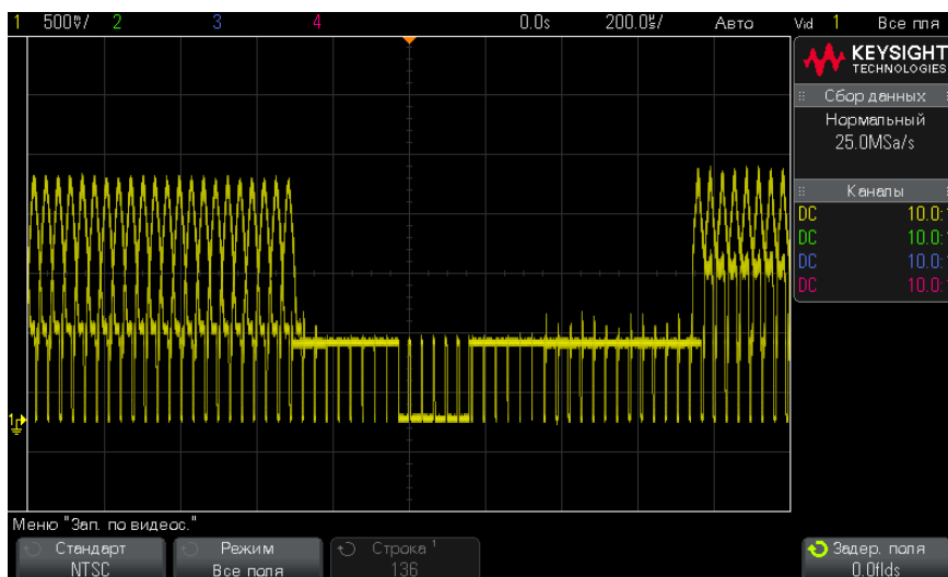
Рис. 30 Запуск по всем полукадрам (All Fields)
