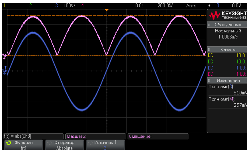
Рис. 12 Пример абсолютного значения
