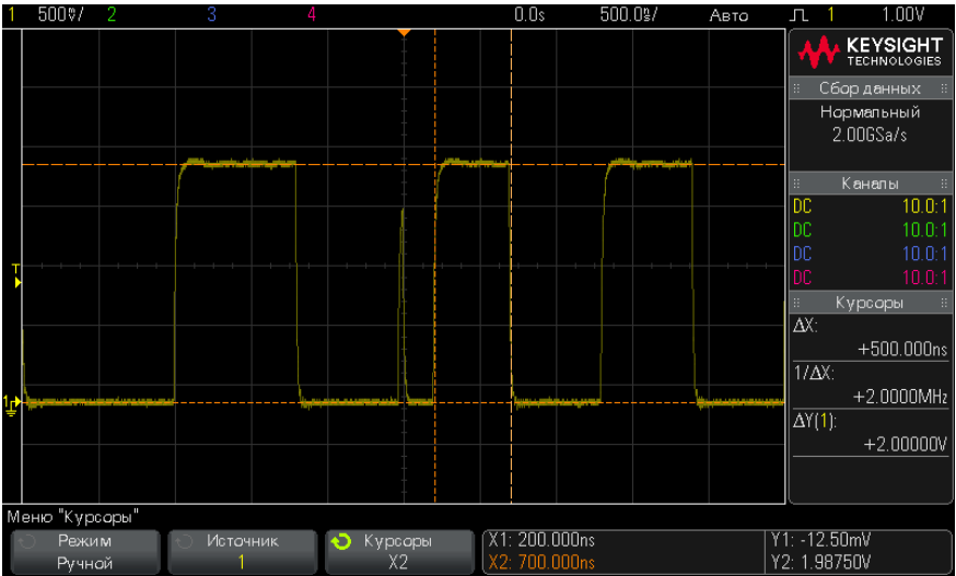
Рис. 43 Измерение длительности импульса с помощью курсоров
