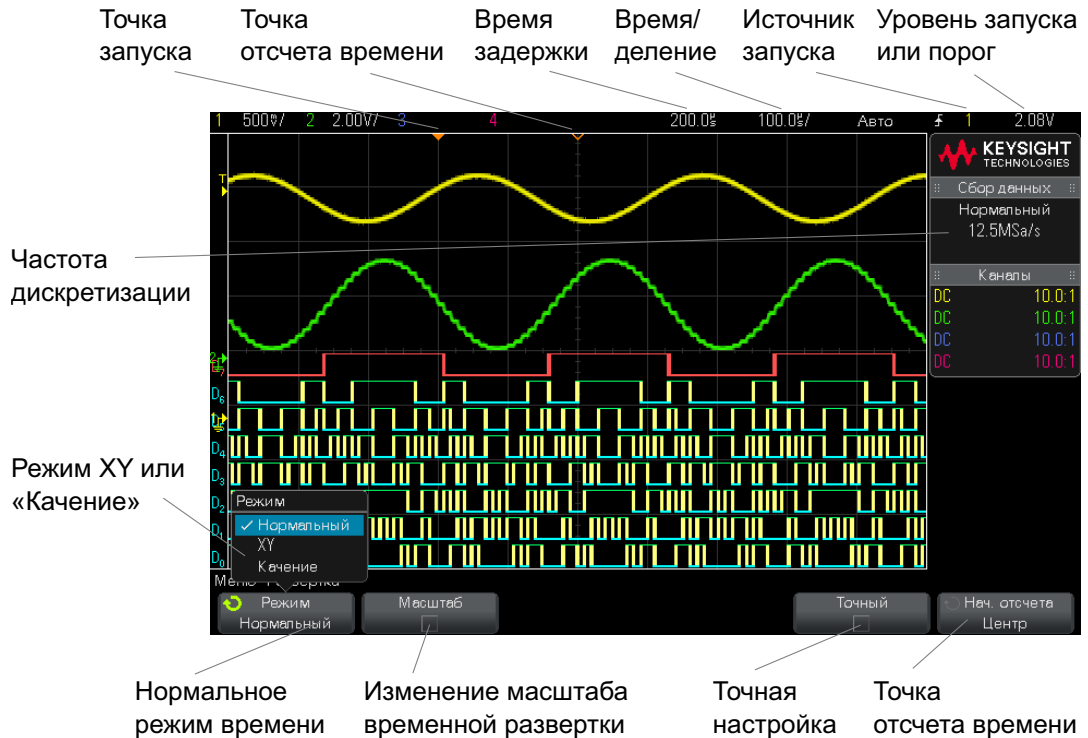
Рис. 2 Меню "Развертка"
