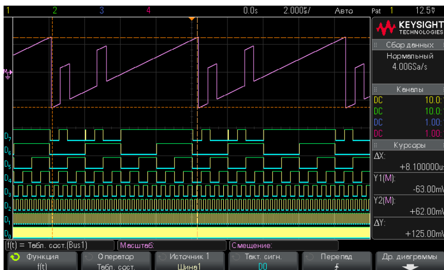
Рис. 19 Пример графика состояния логической шины
