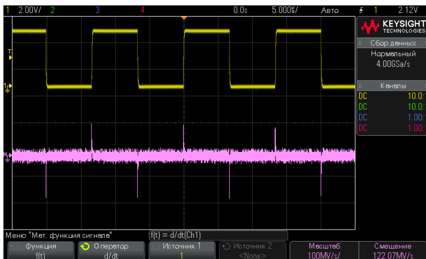
Рис. 7 Пример функции дифференцирования
