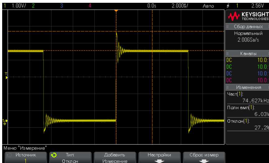
Рис. 46 Автоматическое измерение отклонения от установленного значения
