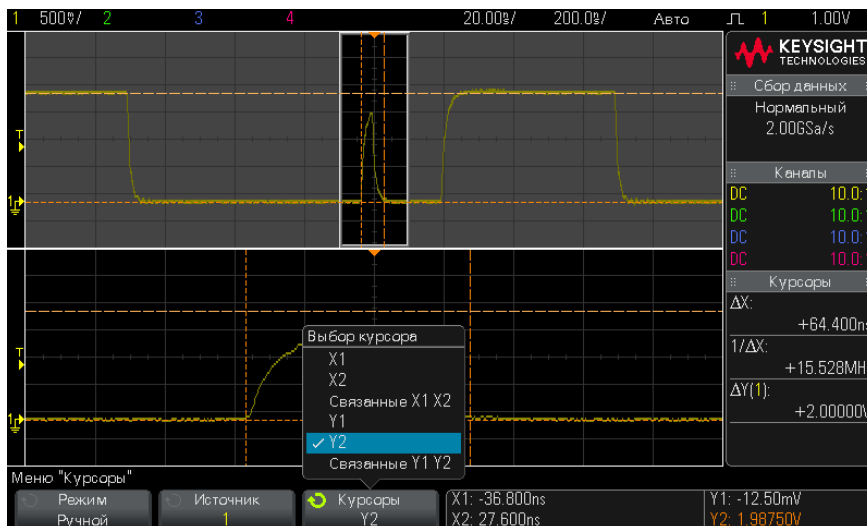
Рис. 42 Курсоры отслеживают окно растянутой развертки
