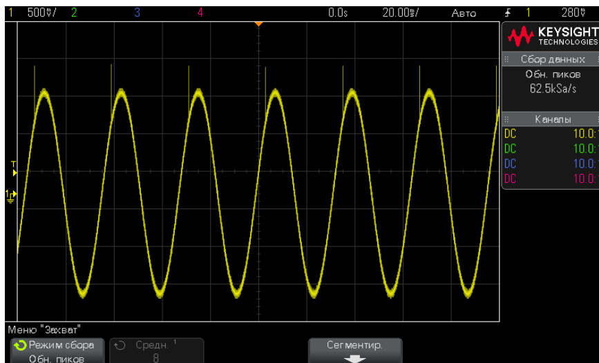
Рис. 37 Синусоида с импульсной помехой, режим обнаружения пиков
